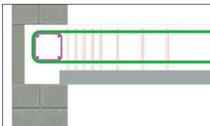
Chaînage 10X10
