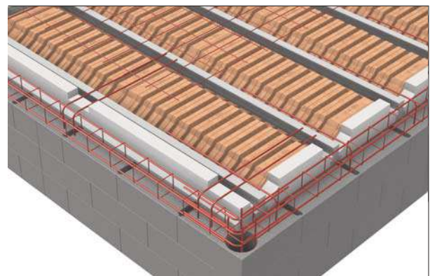
Plancher EBS avec rupteur Total : Stoptherm EB
