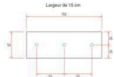
PRELINTEAUX
