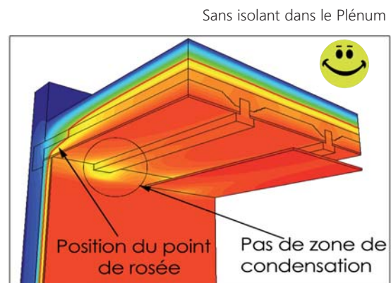
→ Pas de point froid car le Seacbois traite le pont thermique. Les poutrelles sont dans la zone chauffée. Pas de risque de condensation
