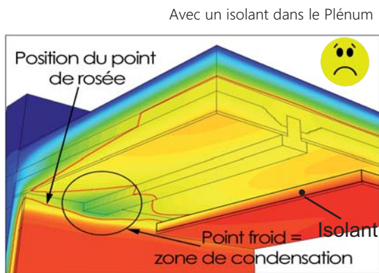
→ Point froid dans le Plénum dû à la présence de l'isolant sous les poutrelles. Risque de condensation à la jonction mur/plancher
