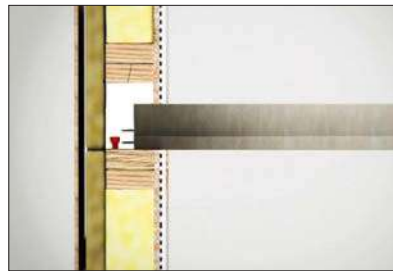
Pose des poutrelles sur le mur
