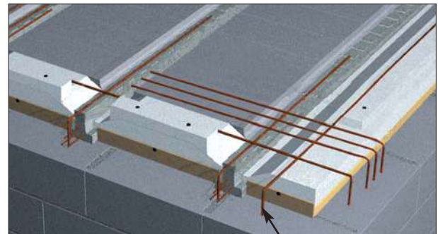
Armatures complémentaires
