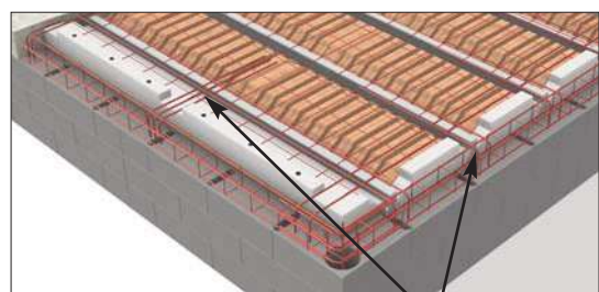
Armatures complémentaires
