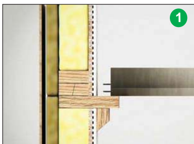
Pose des poutrelles sur corbeaux
