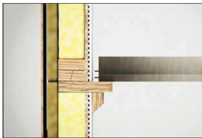
Pose des Poutrelles sur corbeaux
