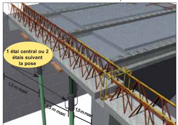
Poutre plate PP 12 x 6 cm
