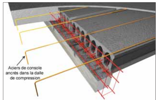
P. à F. dans le prolongement des dalles, montage avec table
