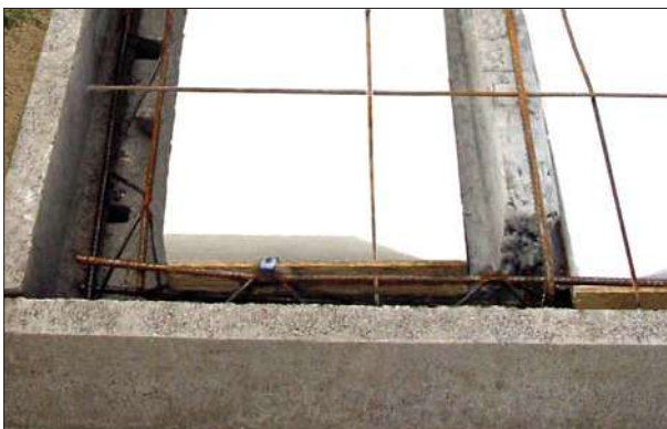
Plancher Hourdis Seacbois Rupteur Partiel : Stoptherm ES
